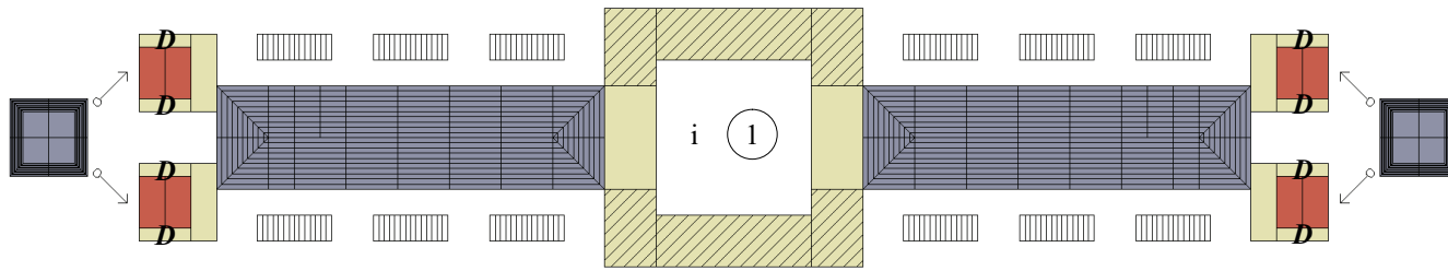
l (1)
