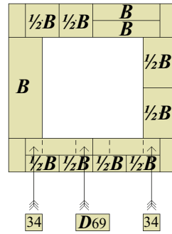
n (1)
